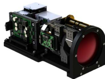
Оптико-электронный тепловизионный модуль для диапазона спектра 3\text{--}5 \text{ мкм} на основе отечественного МФПУ формата 640 \times 512 элементов
