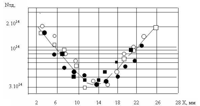
Рис. 1. Распределение термодоноров в p-Si после ВТО в кислороде при 1150^\circ\text{C} в течение 15 минут.
