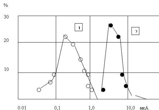
Рис. 6. Распределение темновых токов фотодиодов, содержащих различные концентрации переходных металлов. 1- геттерирование, 2- без геттерирования.
