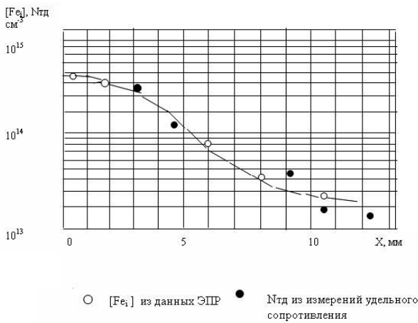
Рис. 3. Сравнение распределений концентраций Fe^0 и термодоноров, полученных из данных ЭПР и измерений удельного сопротивления соответственно.
