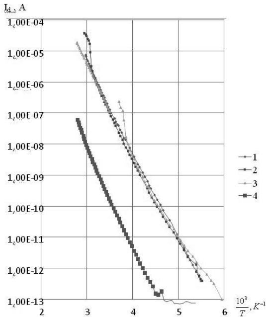
Рис. 4. Температурные зависимости темновых токов кремниевых фотодиодов (ФД). 1, 2, 3 — p-i-n ФД из различных партий (площадь 160 \text{ мм}^2 , кремний p -типа с уд. сопротивлением 10^4 \text{ Ом}\cdot\text{см} ), 4 — p^+-n ФД (площадь 4 \text{ мм}^2 , кремний n — типа с уд. сопротивлением 20 \text{ Ом}\cdot\text{см} )
