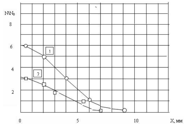
Рис. 2. Профили распределения межузельного железа Fe_i^0 в кремнии после ВТО в течение различного времени: 1 — ВТО при 1150^\circ\text{C} в атмосфере азота, 180 мин. 2 — ВТО при 1150^\circ\text{C} в атмосфере кислорода, 150 мин.
