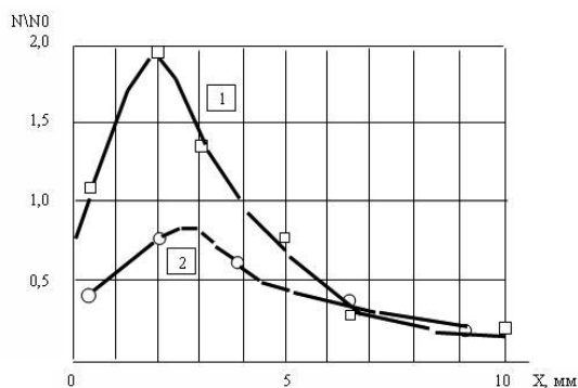
Рис. 5. Распределения Fe^0 по оси слитков, прошедших следующие термообработки: 1 — ВТО при 1150^{\circ}C в атмосфере кислорода с добавкой хлора, 2 — ВТО при 1150^{\circ}C в атмосфере кислорода с последующим геттерированием n+ -слоем фосфора. N_0 = 1.10^{14} \text{ см}^{-3}
