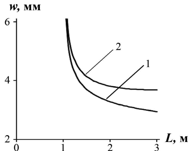
Рис. 2. Графики зависимости диаметров каустик на зеркалах R_1 = -13\text{ м} (кривая 1) и R_2 = 14\text{ м} (кривая 2) от длины L выпукло-вогнутого резонатора.
