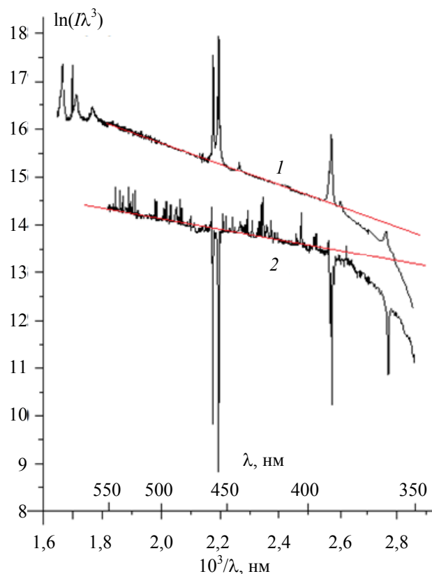
Рис. 2. Спектры цезиевого ИПР лампы с длиной плазменного канала L = 22 мм.
